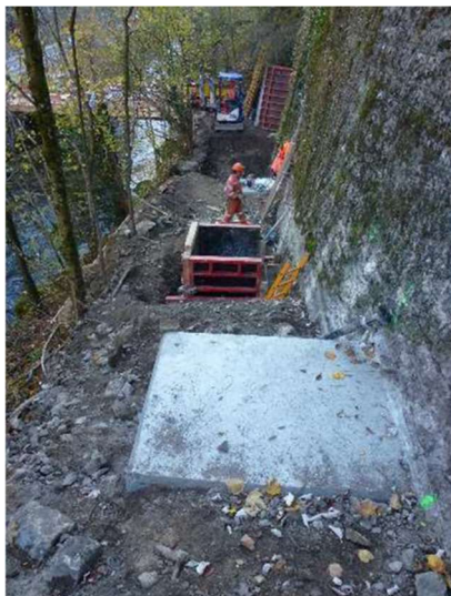
Fondations et Protections montées sur l'échafaudage
