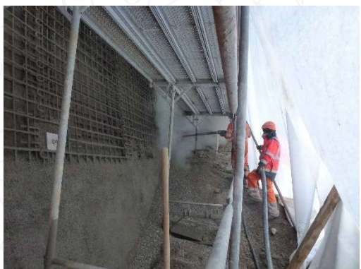
Réalisation du béton projeté aux abords de la rivière depuis l'échafaudage
